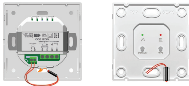
Рис. 7. Подключение датчика температуры воздуха
