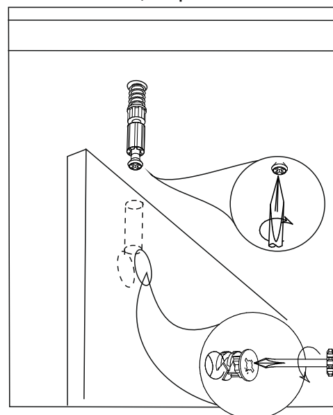
Крепление вязки к боковине эксцентриковой стяжкой
