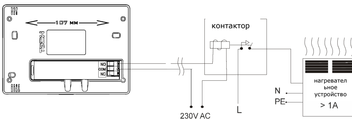
4 Схема подключения регулятора СТ-290 с нагревательным устройством с нагрузкой выше 1А.
