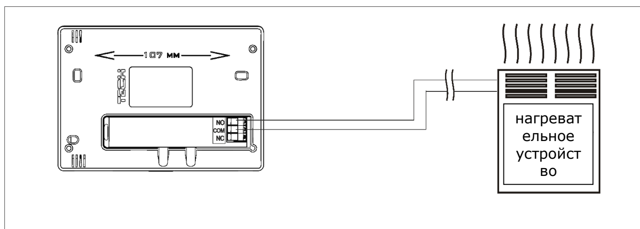
1 Схема подключения регулятора СТ-290 непосредственно с нагревательным устройством.
