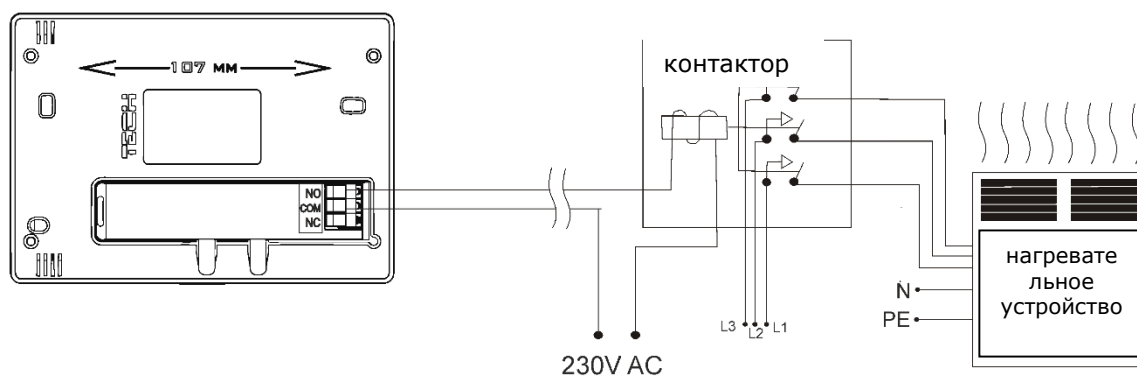
5 Схема подключения регулятора СТ-290 непосредственно с трехфазным нагревательным устройством.
