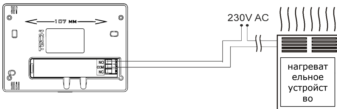
3 Схема подключения регулятора СТ-290 с нагревательным устройством с нагрузкой до 1А.
