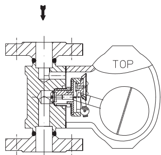
Вертикальное положение (стандарт): Подвод сверху
