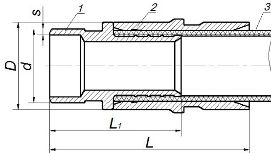
Рис. 7. Переход на сварное соединение с монтажной гильзой для труб ИЗОПЭКС-К
