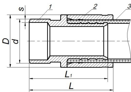
Рис. 6. Переход на сварное соединение с монтажной гильзой для труб ИЗОПЭКС
