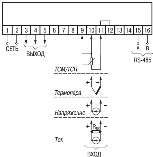
Рисунок В.1 – Общая схема подключения ТРМ201-Н, Щ1, Щ2
