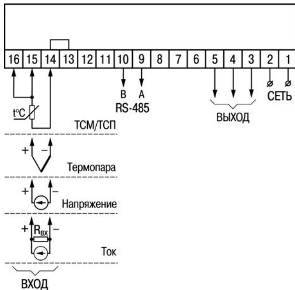
Рисунок В.2 – Общая схема подключения TRM201-N2
