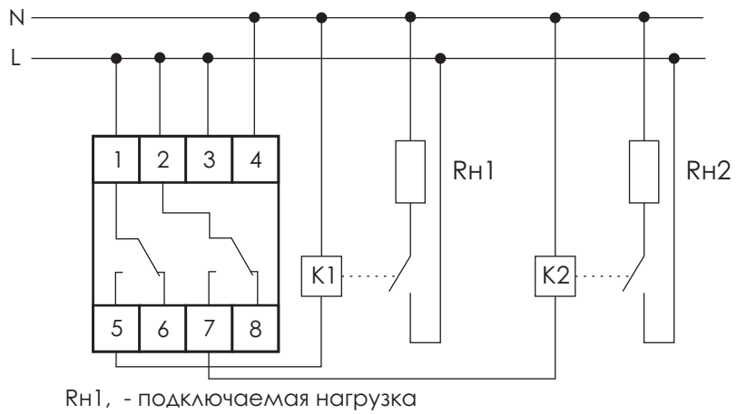
Рис.4 Схема подключения изделия с использованием контактора ток нагрузки более 16А.
