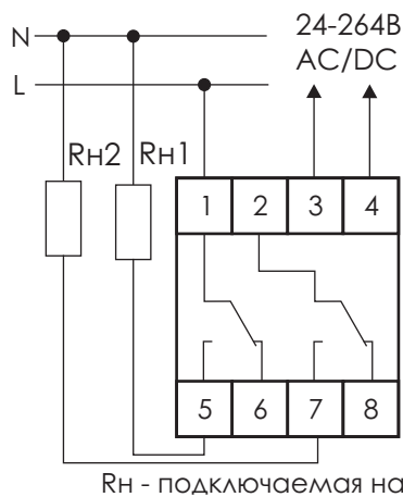
Рис.5 Схема подключения изделия и нагрузки, питающейся, от сети 230В.
