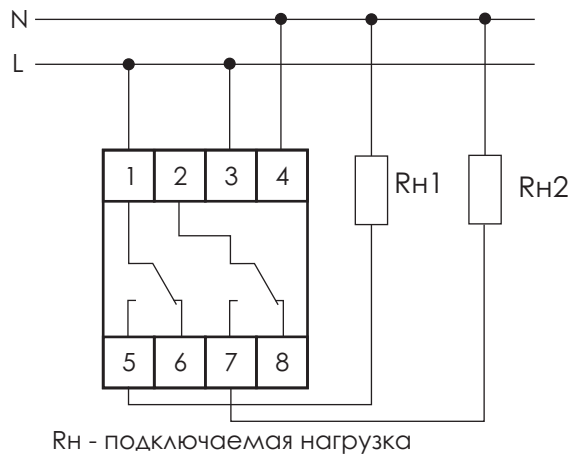
Рис.3 Схема подключения изделия и нагрузки к сети 230В.
