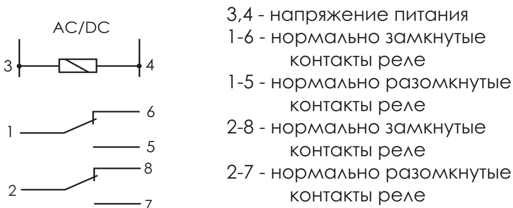
Рис.2 Назначение контактов.
