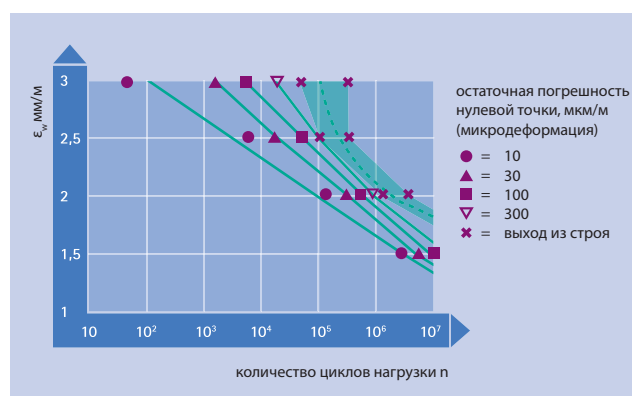
Пример графика, описывающего усталостную долговечность тензорезисторов
