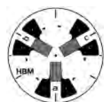
розетка 0^\circ/60^\circ/120^\circ например, RY7x
