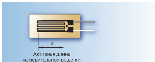
Схема тензодатчика
