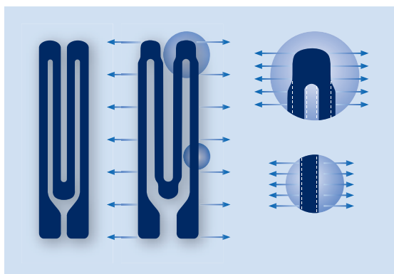
Иллюстрация поперечной чувствительности измерительной решетки
