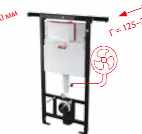
AM102/1120V Jádromodul Скрытая система инсталляции с возможностью вентиляции для сухой установки – при реконструкции ванных комнат в панельных домах
