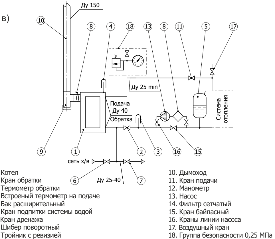
Рис. 6 Рекомендуемые схемы подключения котла
