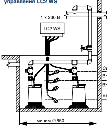
Стационарная установка с двумя насосами и шкафом управления LC2 WS
