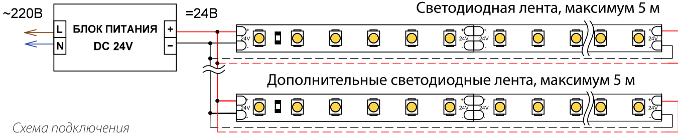
Схема подключения
