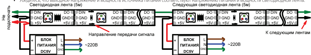
Рис.1. Схема подключения ленты без использования внешнего контроллера (максимум 1024 пикселя, общий рисунок динамического эффекта при переходе с ленты на ленту сохранятся).
