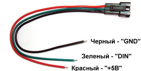
Рис.3. Кабель для подключения открытой ленты и ленты с индексом «SE»
