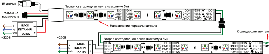
Рис.1. Схема подключения ленты без использования внешнего контроллера (на примере лент с негерметичными разъемами)
