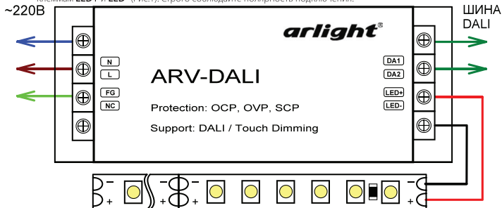
Рис.1. Подключение источника напряжения
