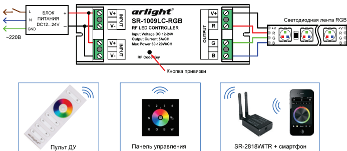
Рис.2. Схема подключения оборудования на примере контроллера SR-1009LC-RGB.
