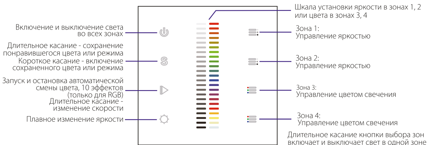
Рис.4. Назначение сенсорных кнопок
