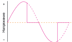
Диммирование по заднему фронту (Trailing edge dimming)
