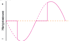
Диммирование по переднему фронту (Leading edge dimming)
