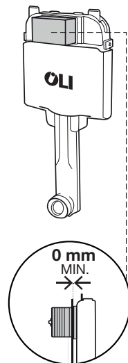
OLI74 PLUS
