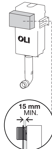
QUADRA PLUS
