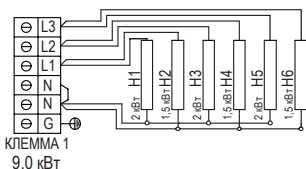
Рис. 5. Электрическая схема
