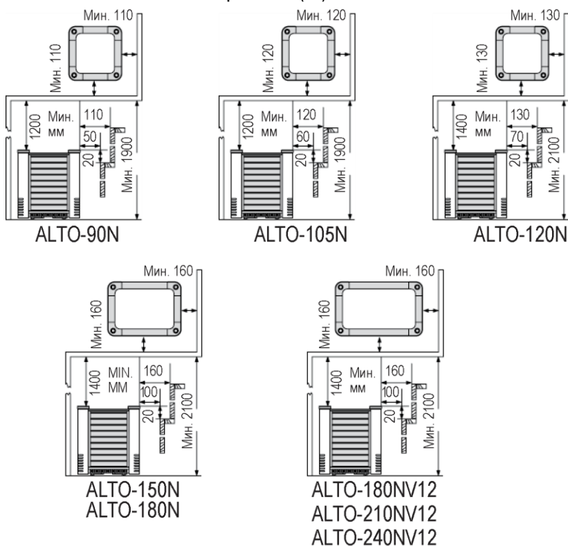
Рис. 2. Минимальные безопасные расстояния (мм)
