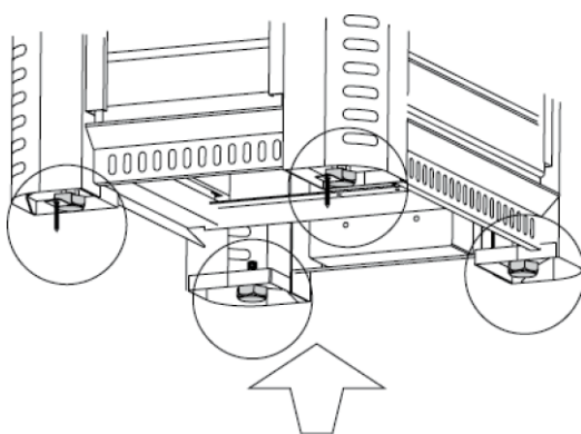
Рис. 1. Установка
