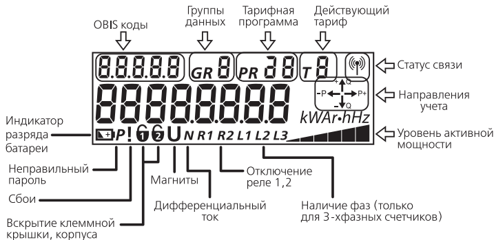
Рисунок 2.2 – Информация, выводимая на ЖКИ счетчика
