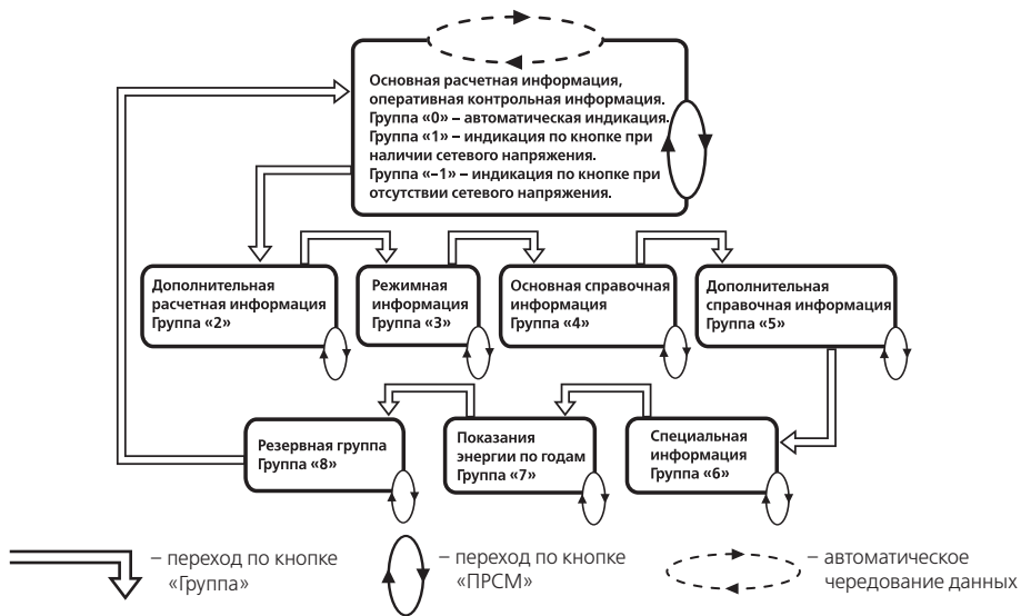
Рисунок 2.3 – Алгоритм переключения основных групп режимов индикации в счетчике
