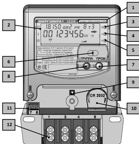
Рисунок 2.1 – Внешний вид счетчика
