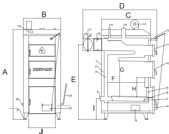
Oznaczenia rysunku technicznego
