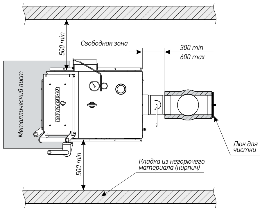
Рисунок 6 Схема установки котла
