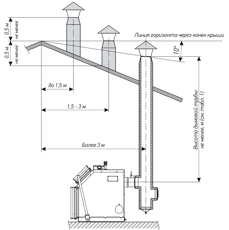
Рисунок 8 Схема установки дымовой трубы
