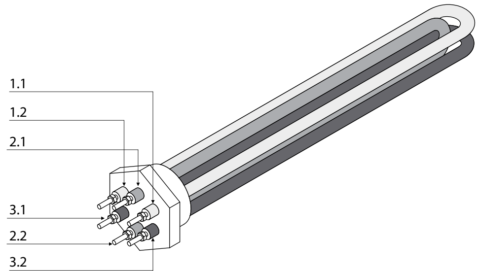
Рисунок 3. Блок ТЭН
