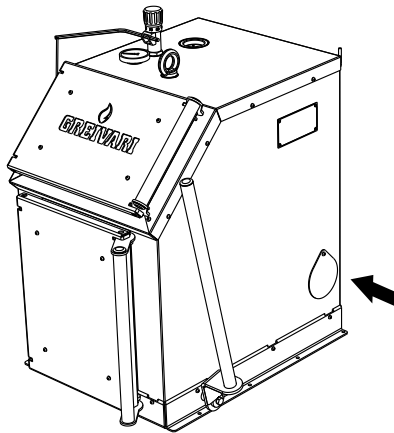
Рисунок 5. Место подключения блока ТЭН к котлу «Адмирал»
