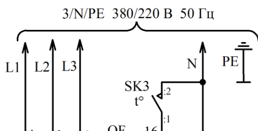
Рисунок 1 – Электроводонагреватель аккумуляционный с термоизоляцией ЭВА.
