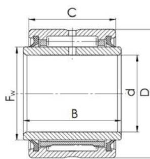
NA 49 2RS
