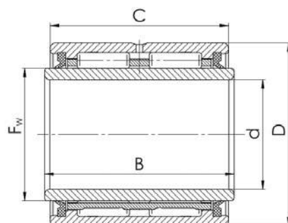
NA 69 2RS
