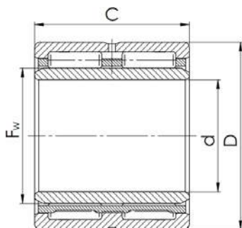
NA69
