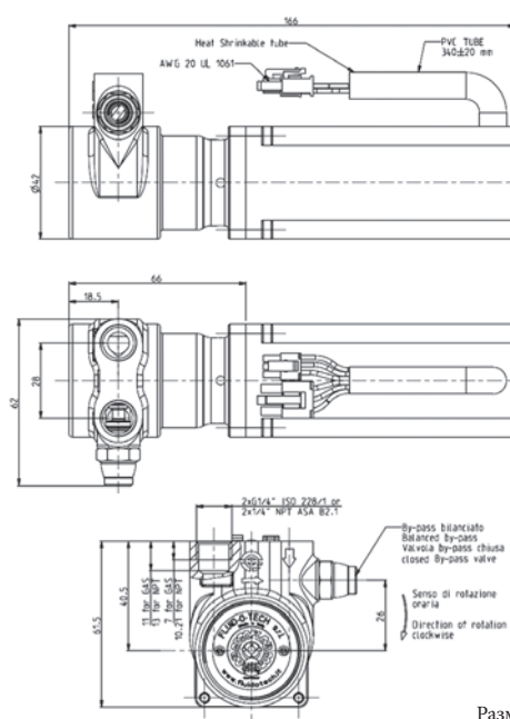
GA0072 - двигатель без щеток 90-93-02
