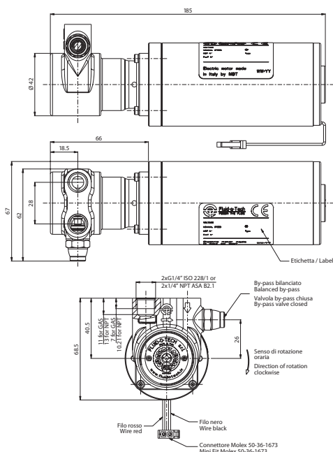
GA0072 - двигатель со щетками D56 H102 90-54-37
