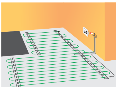
Установка теплого пола в бухте
