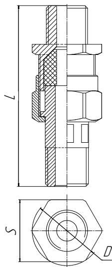
габаритный чертеж
