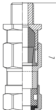
габаритный чертёж
