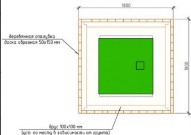
Вид сверху
