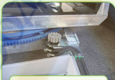
ГИДРАВЛИЧЕСКИЙ ПРИВОД ПОВОРОТА ПЛАТФОРМЫ
