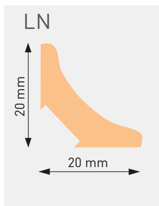
PROFIL NAROŻNY
