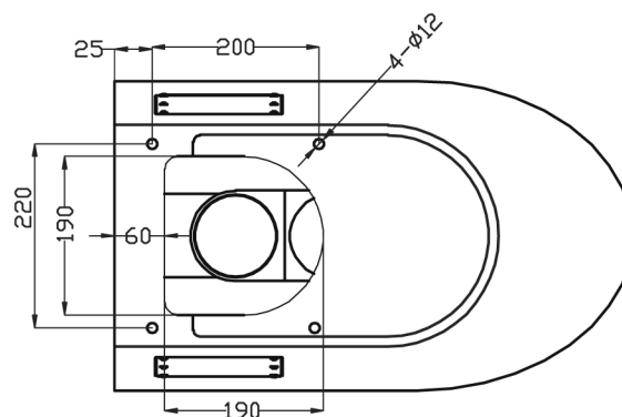
ВИД СНИЗУ
