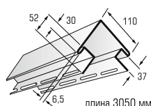
2 наружный угол
