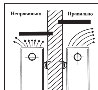
Рис. 5.3. Схема установки радиатора под подоконником
