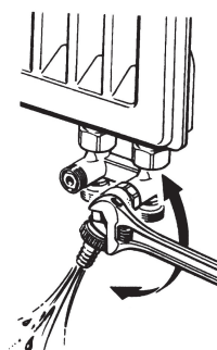
Рис. 5.5. Дренаж Радиатора
