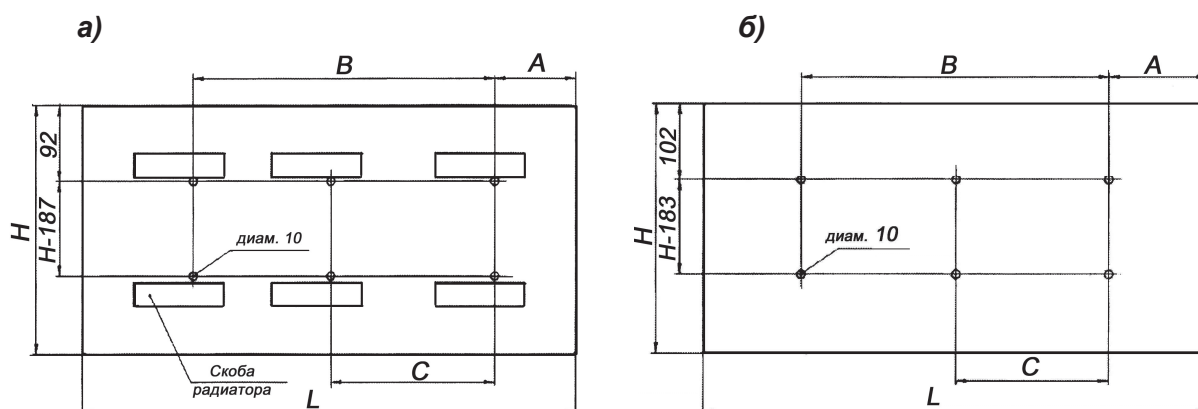
Рис. 5.2. Разметка мест установки кронштейнов радиаторов: а – «PRADO Classic» всех типов и «PRADO Universal» типов 10 и 11; б - «PRADO Universal» типов 20, 21, 22, 30 и 33
