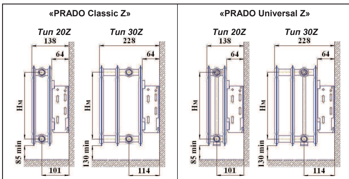
Рис. 1.4. Общий вид и габаритные размеры гигиенических радиаторов «PRADO»
