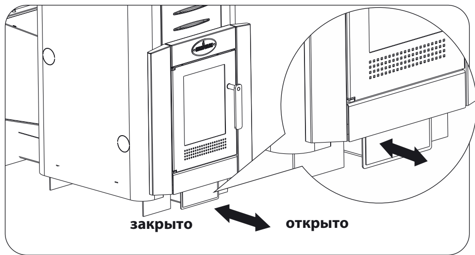
Рисунок 7. Регулировка тяги с помощью шибера
