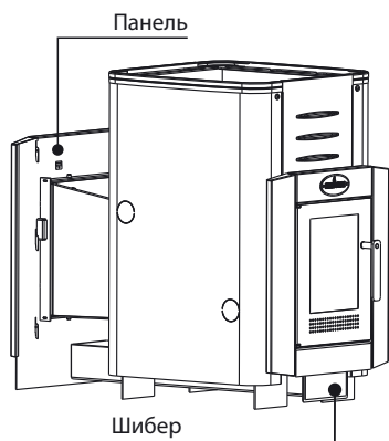
Рисунок 2. Печь Кирасир Шведка. Вид сзади
