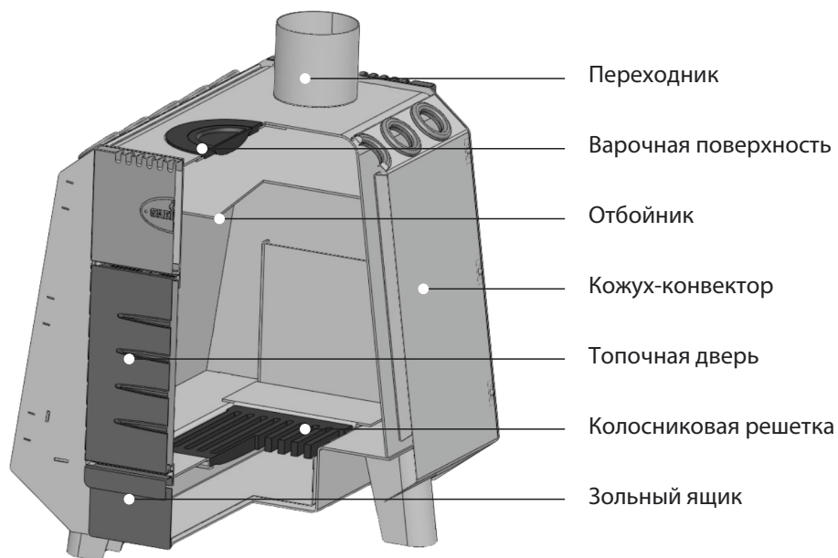
Рисунок 1. Конструкция печи Комбат (вид спереди)
