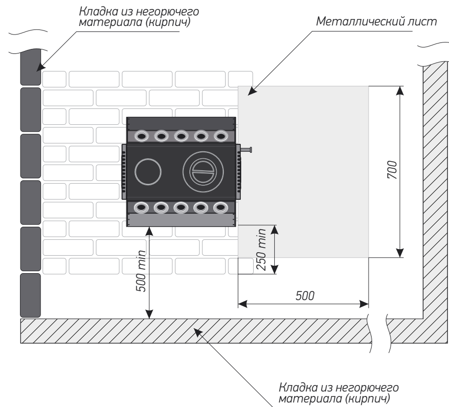
Рисунок 3. Схема установки печи (вид сверху)
