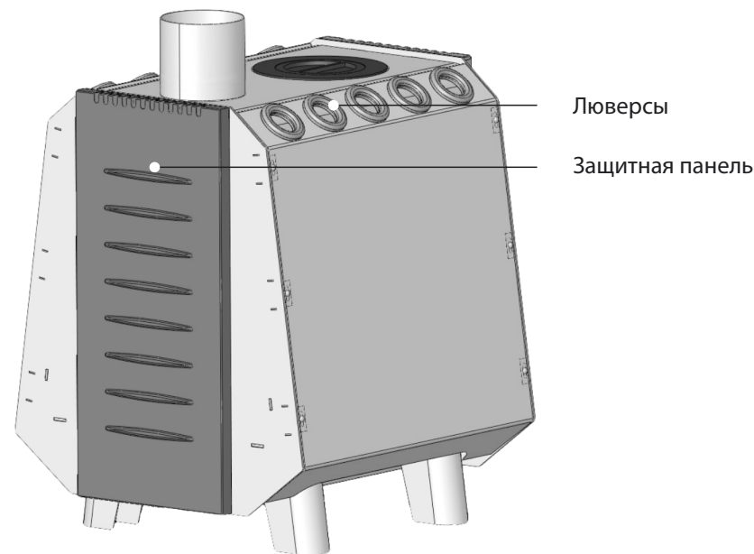
Рисунок 2. Конструкция печи Комбат (вид сзади)
