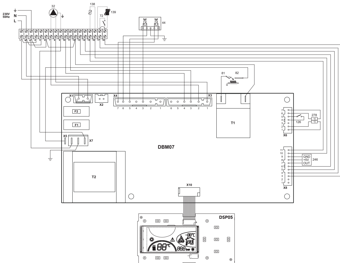
рис. 25 - Электрическая схема
