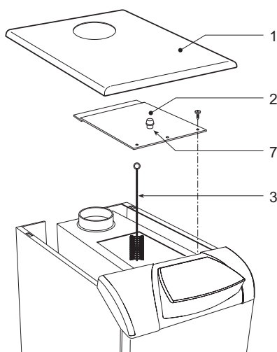
рис. 20 - Очистка котла
