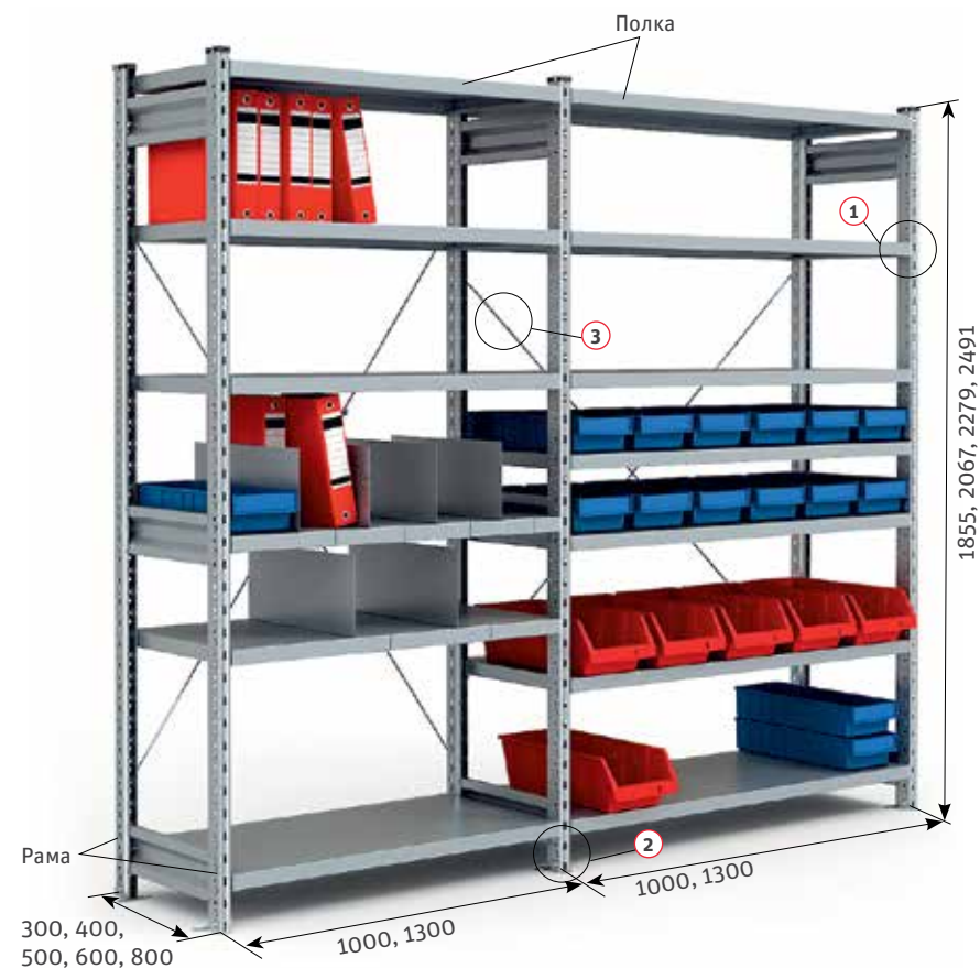
Стеллаж СТ-031 (2 секции)
