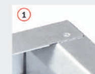
Жесткая заделка угла (Clinch) и завальцовка краев полки
