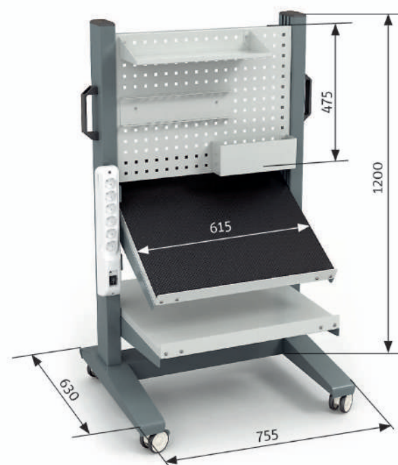
Стойка подкатная ДиКом CP-021 ESD
