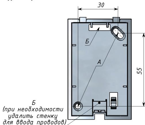
Рисунок 2 – Основание корпуса - разметка крепления извещателя
