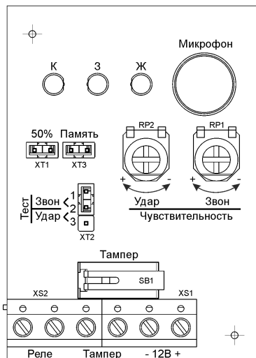
Рисунок 1 - Внешний вид платы извещателя
