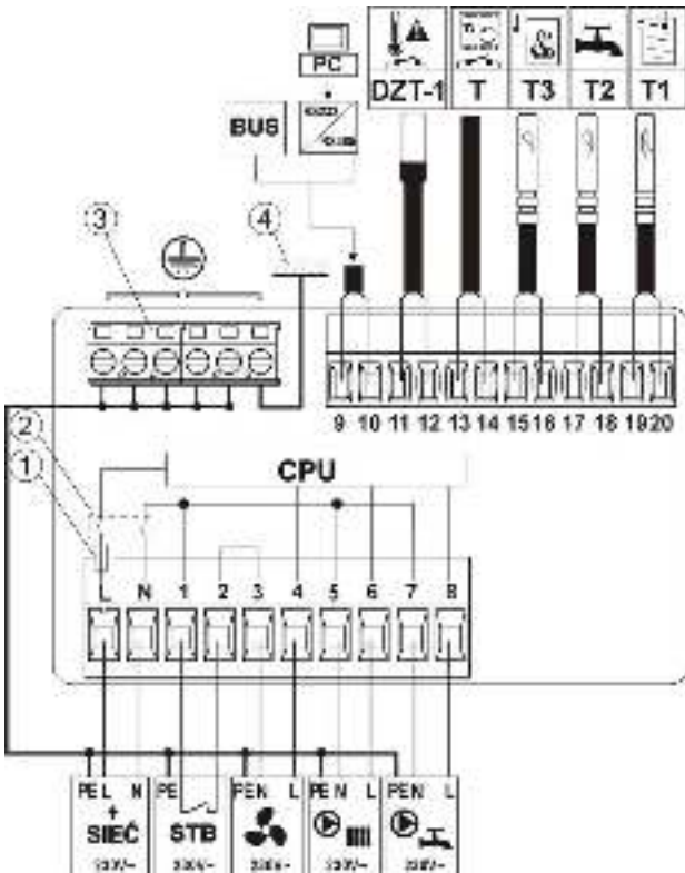
Рис. 11 Схема электрических соединений с внешними устройствами, версия ST. где: T1 – датчик температуры котла (тип СТ4), T2 – датчики температуры тёплой воды (тип СТ4), T3 – датчик температуры выхлопных газов (тип СТ2s, СТ2s-2), T – комнатный термостат, DZT-1 – дополнительная термическая страховка (тип DZT-1 85°C или 90°C), RS232/RS485 –преобразователь, BUS – соединение цифровой коммуникации с компьютером (опция), 1 – сетевой предохранитель в регуляторе, 2 – сетевой выключатель в регуляторе, 3 – охранные зажимы PE, 4 – металлический корпус регулятора, СЕТЬ – сетевой провод, STB – ограничитель температуры безопасности,
