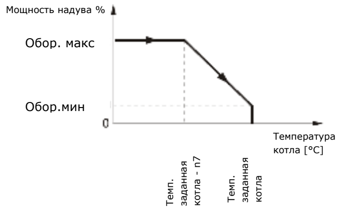
Рис. 17 Снижение оборотов вентилятора при классической регуляции
