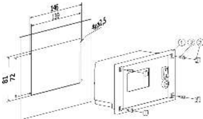
Рис. 8 Установка регулятора в монтажной доске, где: 1 – регулятор, 2 – винт 2.9x9, 3 – заглушка.
