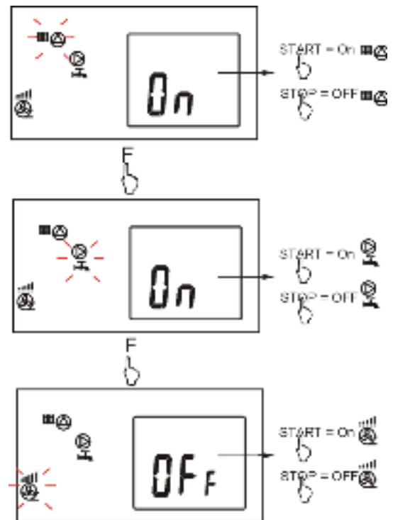
Рис. 5 Ручное управление
