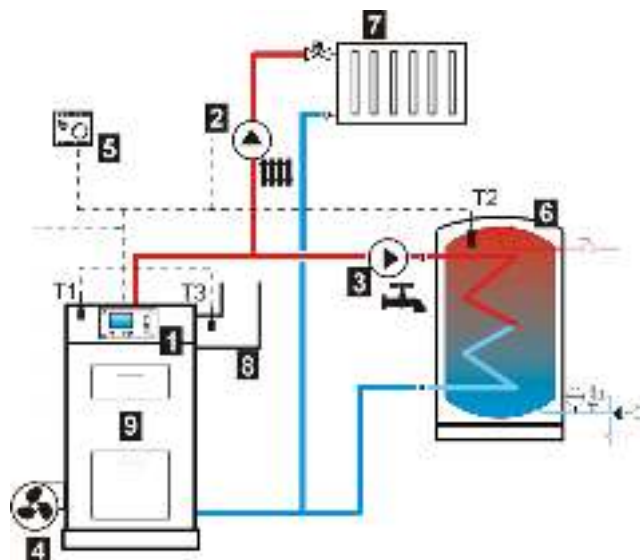
Рис. 6 Обслуживаемая регулятором гидравлическая схема, где: 1 – регулятор, 2 – насос центрального обогрева, 3 – насос тёплой воды, 4 – вентилятор, 5 – комнатный термостат, 6 – бак тёплой воды, 7 – установка центрального обогрева, 8 – дымоход, 9 – котёл, T1 – датчик температуры котла, T2 – датчик температуры тёплой воды, T3 – датчик температуры выхлопных газов (как опция, не требуется для нормальной работы).
