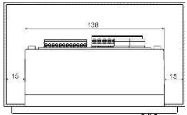
Рис. 10 Условия застройки регулятора
