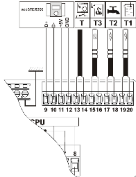
Рис. 12 Схема электрических соединений с внешними устройствами, версия ES. где: T1 – датчики температуры котла (тип СТ4), T2 – датчики температуры горячего водоснабжения (тип СТ4), T3 – датчик температуры продуктов сгорания (тип СТ2s, СТ2s-2), T – стандартный комнатный термостат, TIS TRONIC 297 – комнатная панель с функцией комнатного термостата.
