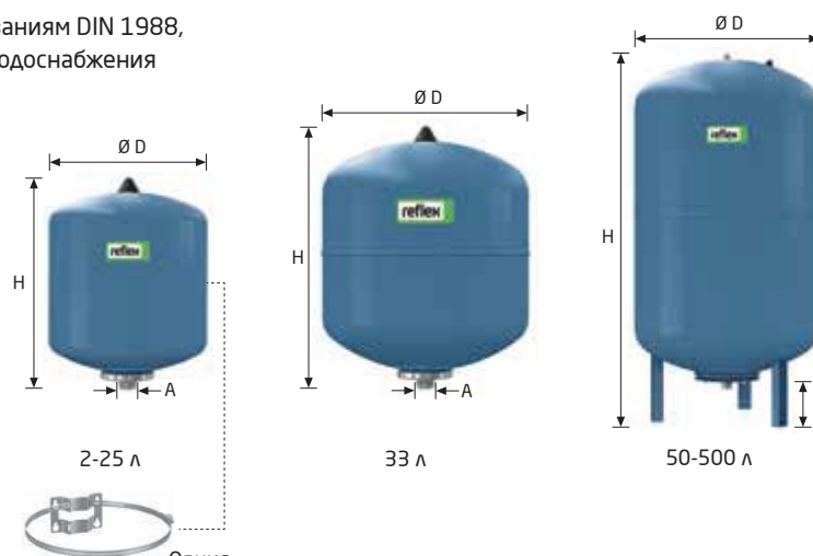
Опция Ленточный хомут для крепления на стене Артикул № 7611000
