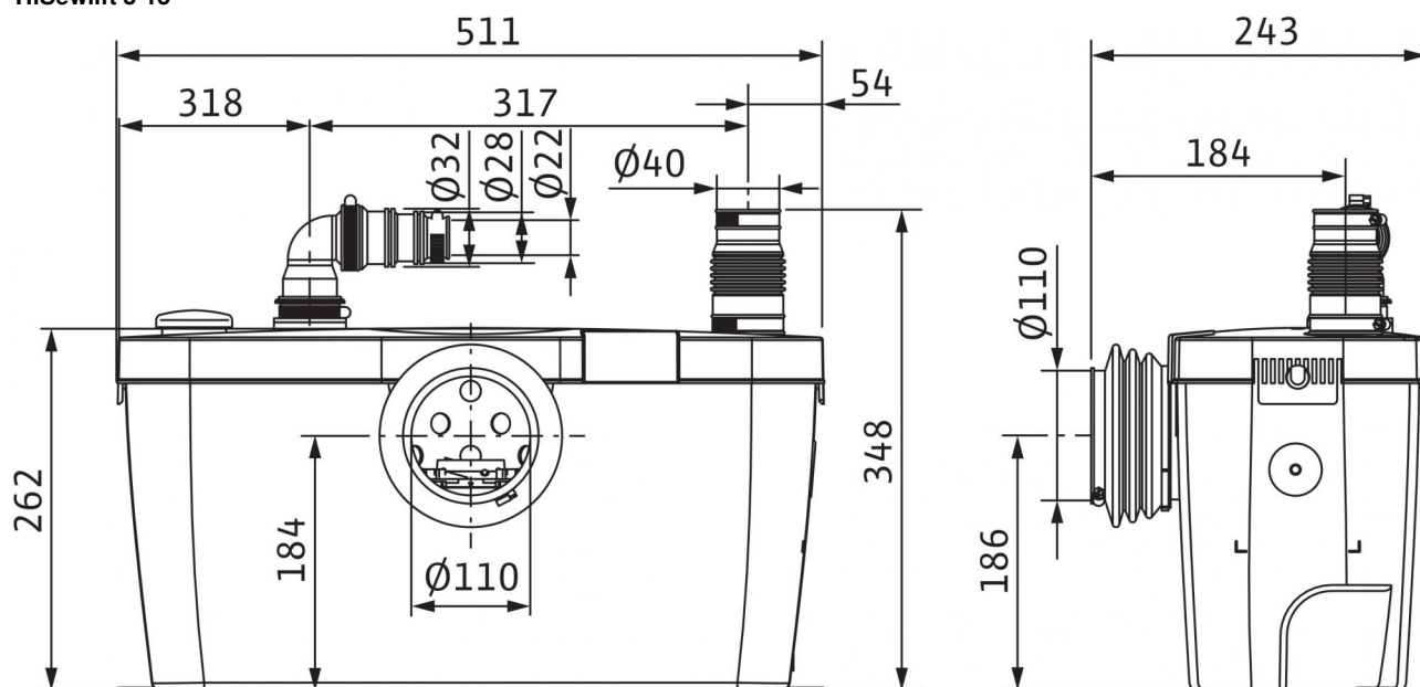
Габаритный чертеж HiSewlift 3-15 HiSewlift 3-15
