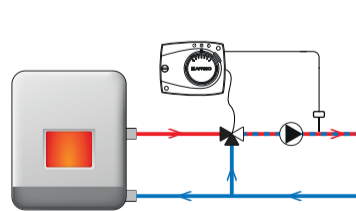
рис. 5 Схемы
