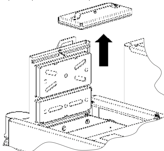
с) вытянуть отбойники
