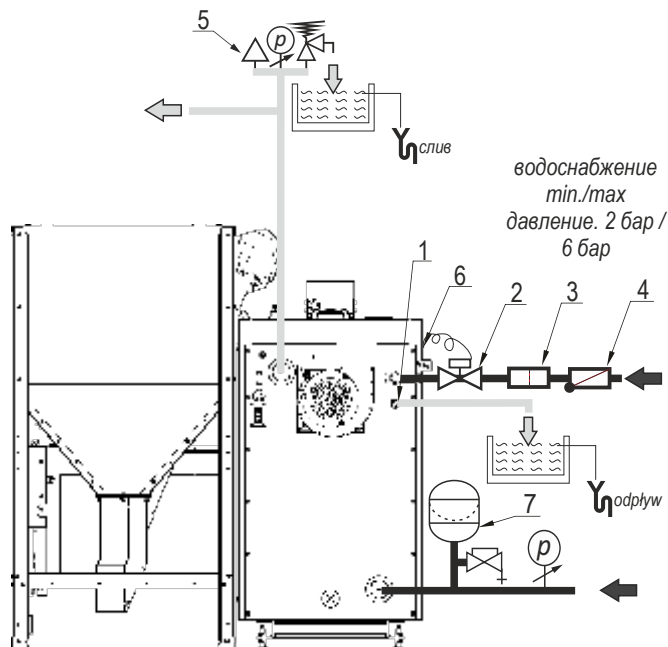
Рисунок 5. Схема примера безопасности котла в закрытой системе::1- спираль; 2-клапан BVTS встроенный в спираль; 3-фильтр воды; 4-обратный клапан; 5-группа безопасности; 6- датчик клапана BVTS; 7- мембранный расширительный бак.
