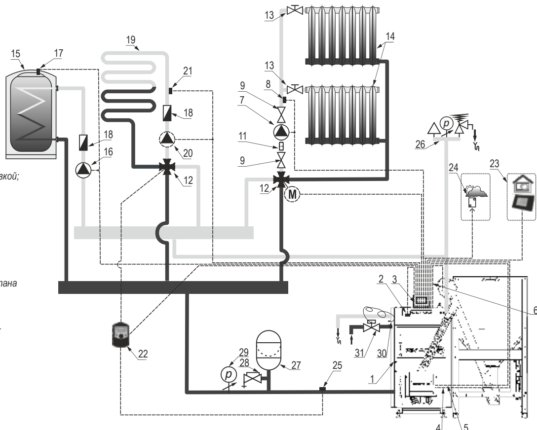
Рисунок 12. Примерная схема отопительной системы закрытого типа с защитой котла от перегрева, реализованная через терморегулятор.
