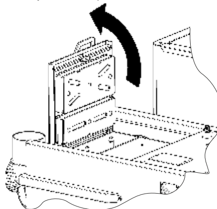
б) открыть верхние очистные двери
