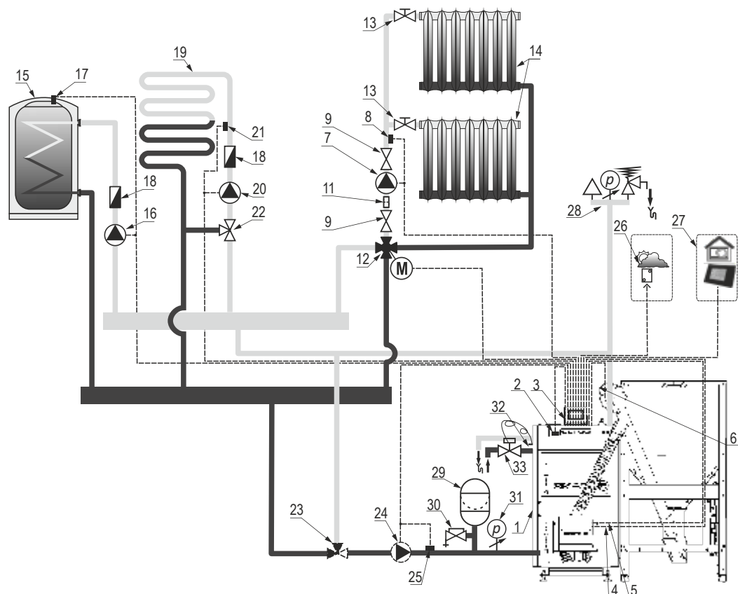
Рисунок 12. Примерная схема отопительной системы закрытого типа с защитой котла от перегрева, реализованная через термостатический клапан.
