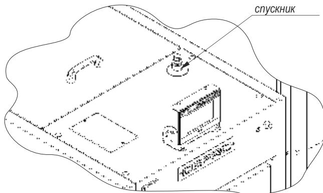
Рисунок 14. Расположение спускника
