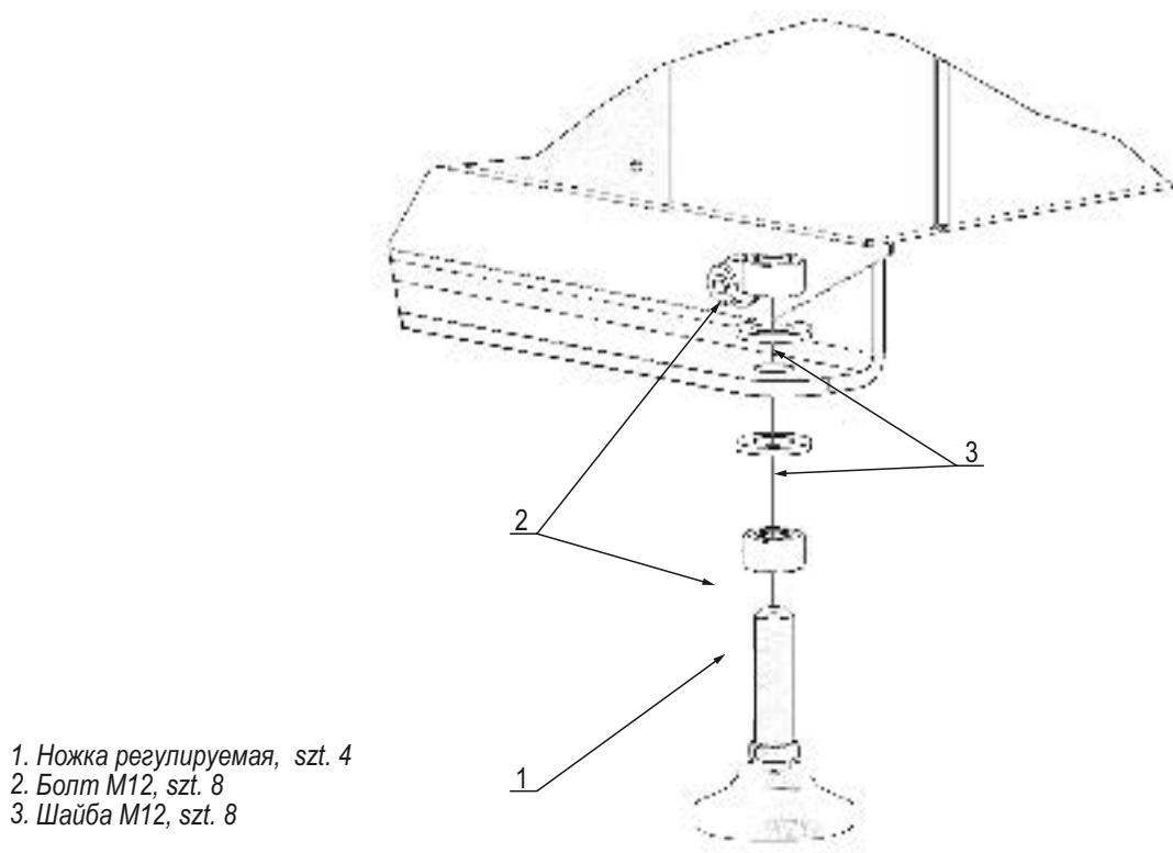
Рисунок 23. Особ монтаж ножек
