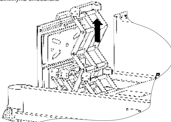
д) вытянуть и очистить экономайзеры; обрат в обратном порядке; проверить правильность сборки
