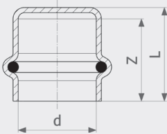
Заглушка Prestabo - не легированная сталь, цинковое гальванированное покрытие Модель 1156
