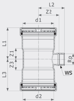
Тройник Prestabo XL - не легированная сталь, цинковое гальванированное покрытие Модель 1117.2XL
