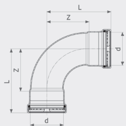
Отвод 90° Prestabo XL - нелегированная сталь, цинковое гальванизованное покрытие Модель 1116XL
