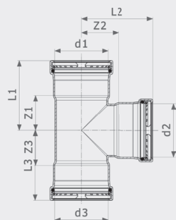
Тройник Prestabo XL - не легированная сталь, цинковое гальванированное покрытие Модель 1118XL
