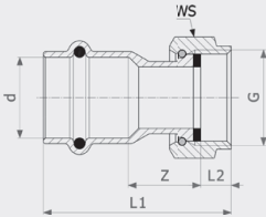
Переход на резьбовые соединения Prestabo - не легированная сталь, цинковое гальванированное покрытие Модель 1163
