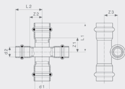
Крестовина Prestabo - не легированная сталь, цинковое гальванизированное покрытие Модель 1148
