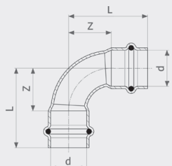
Отвод 90° Prestabo - нелегированная сталь, цинковое гальванизованное покрытие Модель 1116
