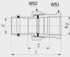
Соединительный элемент резьбовой разъемный Prestabo - не легированная сталь, цинковое гальванированное покрытие Модель 1162
