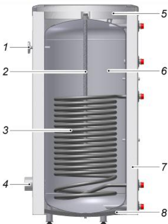
Рис. 1 Разрез водонагревателя W-E хх.81
