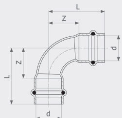
Отвод 90° Prestabo - нелегированная сталь, цинковое гальванизированное покрытие Модель 1116
