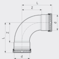
Отвод 90° Prestabo XL - нелегированная сталь, цинковое гальванизированное покрытие Модель 1116XL
