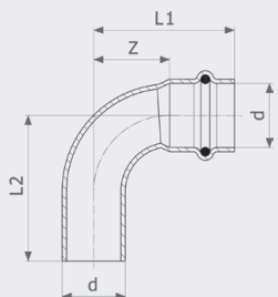
Отвод 90° Prestabo - нелегированная сталь, цинковое гальванизированное покрытие Модель 1116.1
