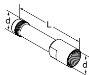
Удлинитель для измерительного штанца M14x1
