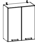
■ Шкаф навесной 600x720x290 мм Ш600
