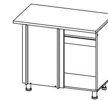
■ Стол под мойку (угловой) 900x850x420 мм Столешн.: 1000x600 мм M1000y
