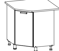
■ Стол под мойку (угловой) 420x850x420 мм Столешн.: 850x850x850 мм М850у
