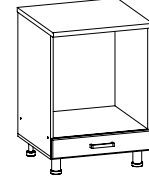
■ Стол-рабочий (под плиту) 600x850x420 мм Столешн.: 600x600 мм С600п
