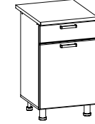
■ Стол-рабочий (с ящиком и створками) 500x850x420 мм Столешн.: 500x600 мм С500яс
