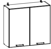
■ Шкаф навесной 800x720x290 мм Ш800
