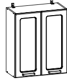
■ Шкаф навесной (со стеклом) 600x720x290 мм Ш600с
