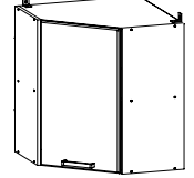
■ Шкаф угловой 600x720x550 мм Ш600у
