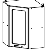
■ Шкаф угловой (со стеклом) 550x720x550 мм Ш550ус
