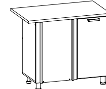
■ Стол под мойку (угловой) Правый 1000x850x420 мм Столешн.: 1000x600 мм М1000у
